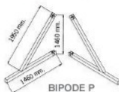
BIPODE P
